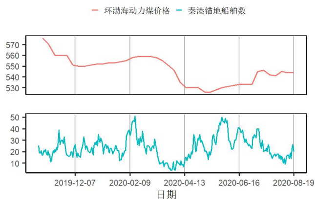
图14 截至2020年08月19日的一周，环渤海动力煤价格周环比维持在544元/吨，秦港锚地船舶均值增加5.71艘至18.86艘
