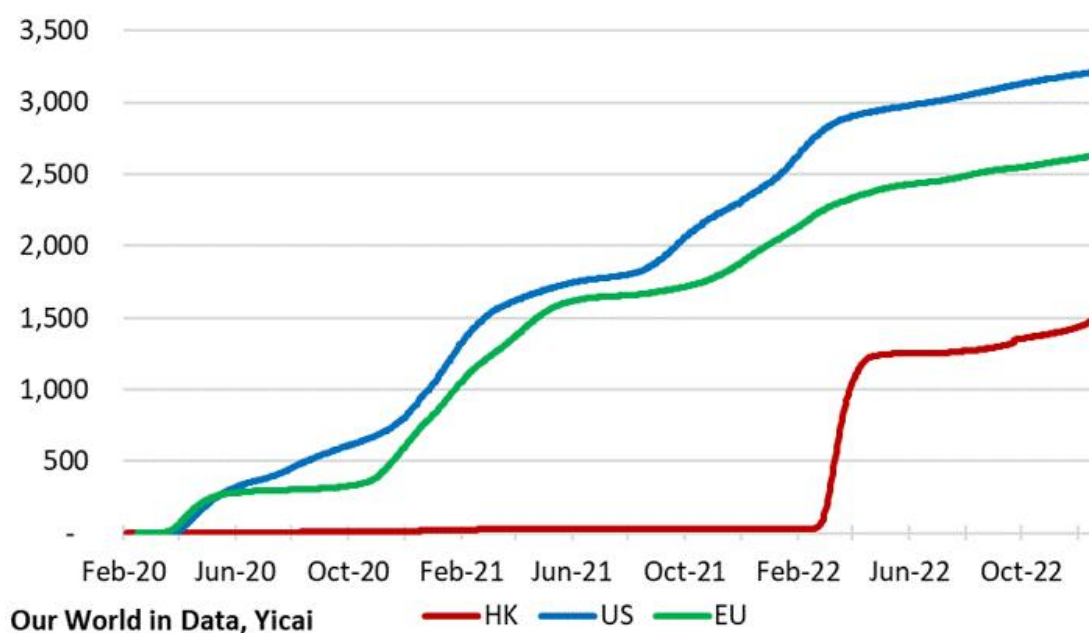
图 1：每百万人口的累计死亡数
